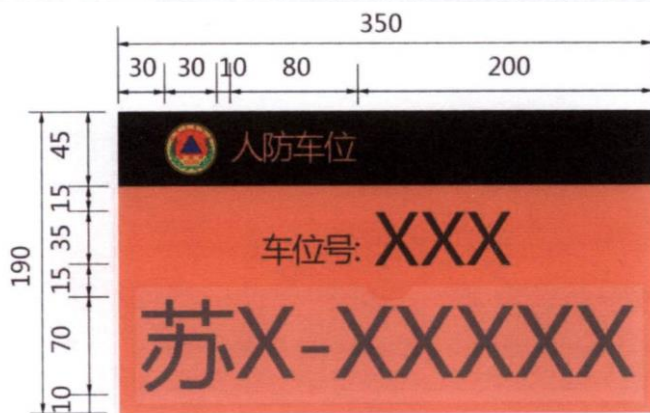
图4 标识牌(小)样式及尺寸示例
