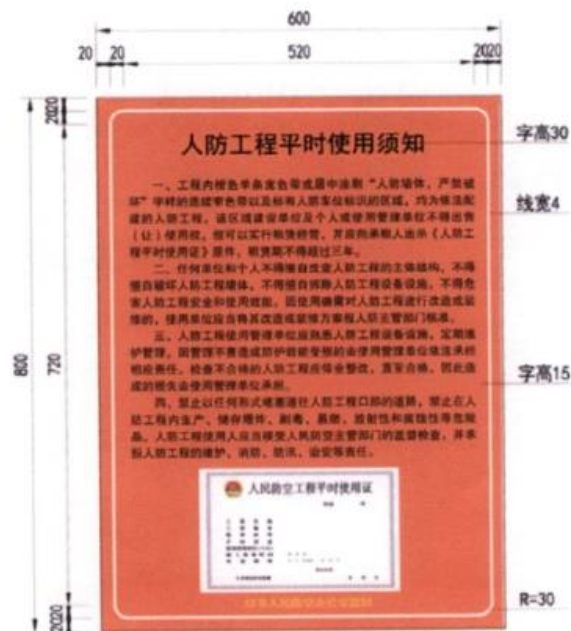
图3 管理标识牌样式及尺寸示例
