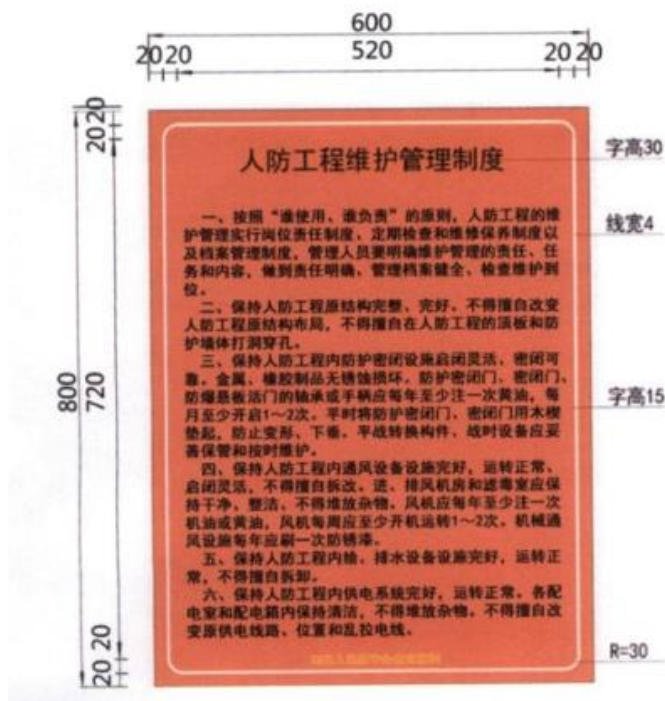
图2 管理标识牌样式及尺寸示例
