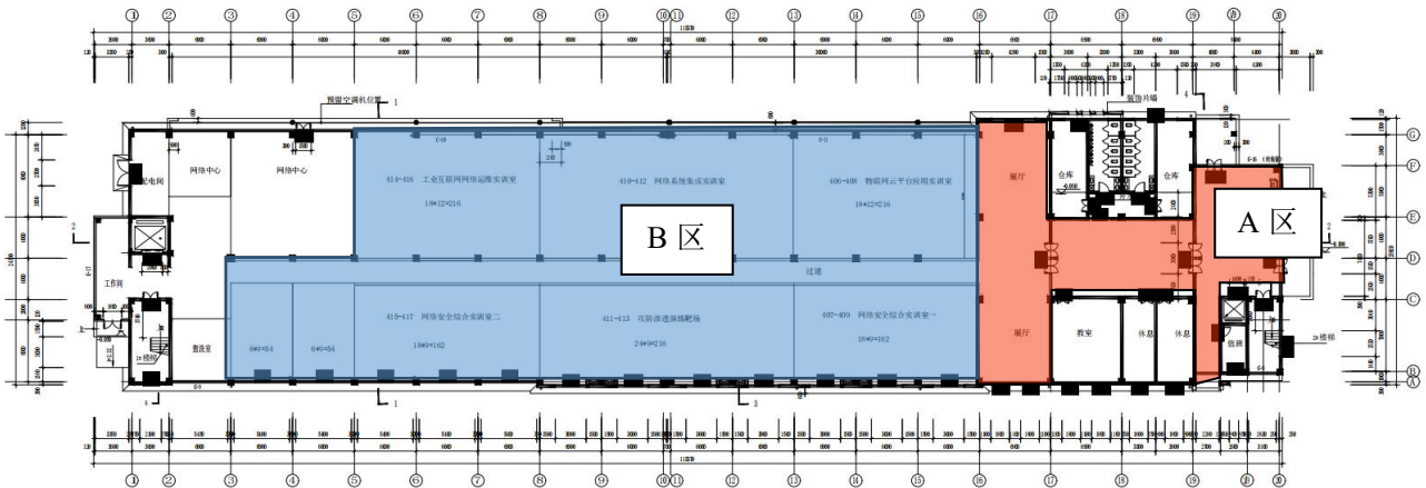
四层平面图
