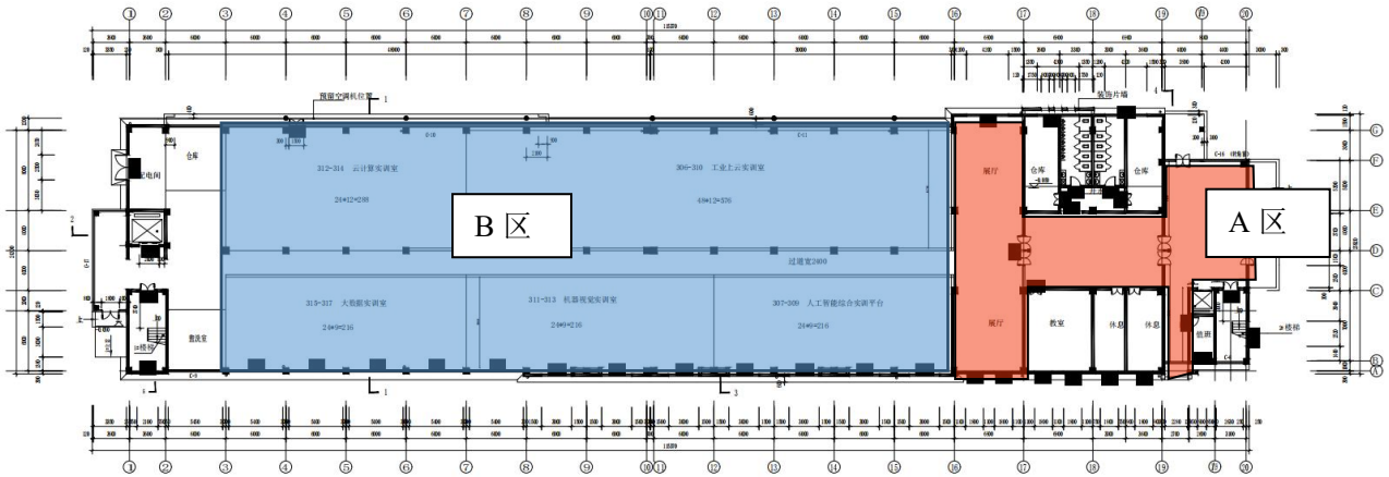
三层平面图
