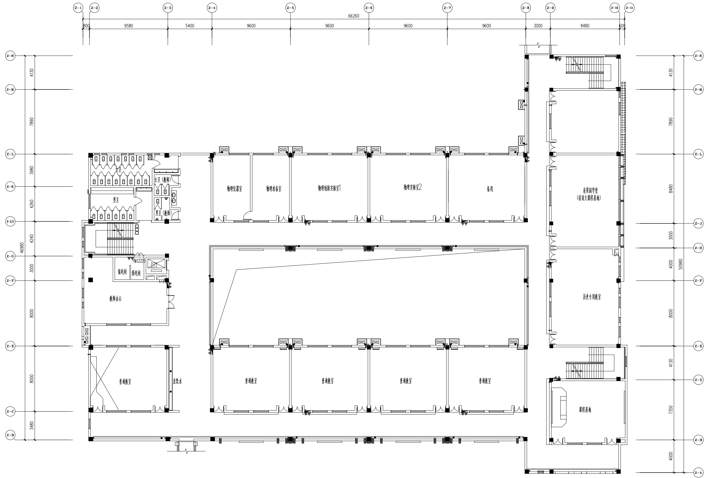
常州市田家炳初级中学1#楼三层平面图
