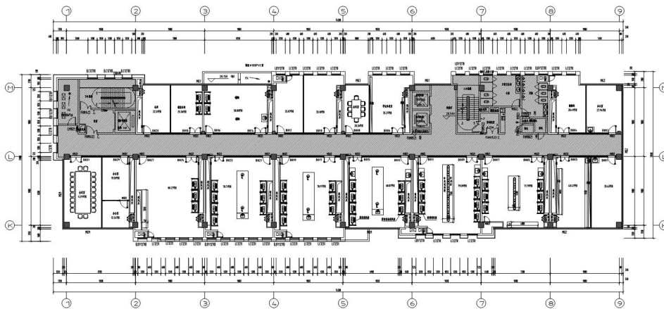
4. 九楼平面图
