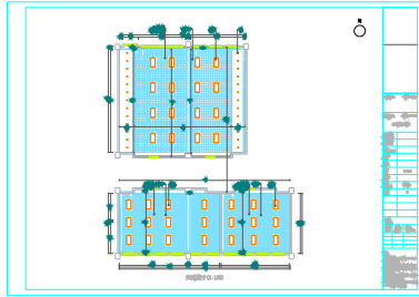
天花灯位图
