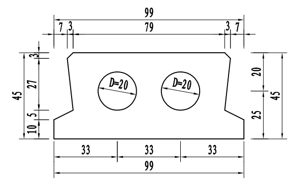
中板
