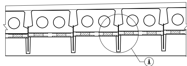
立面图 1:50
