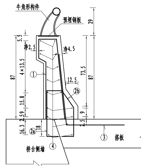
组合式护栏钢筋横断面 1:20
