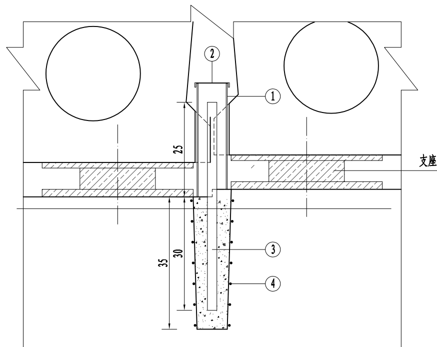
A 大样 1:10
