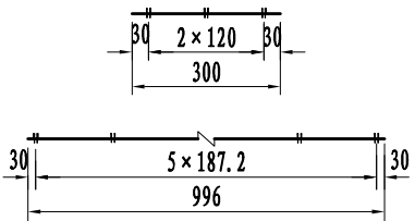
牛角形布置示意图
