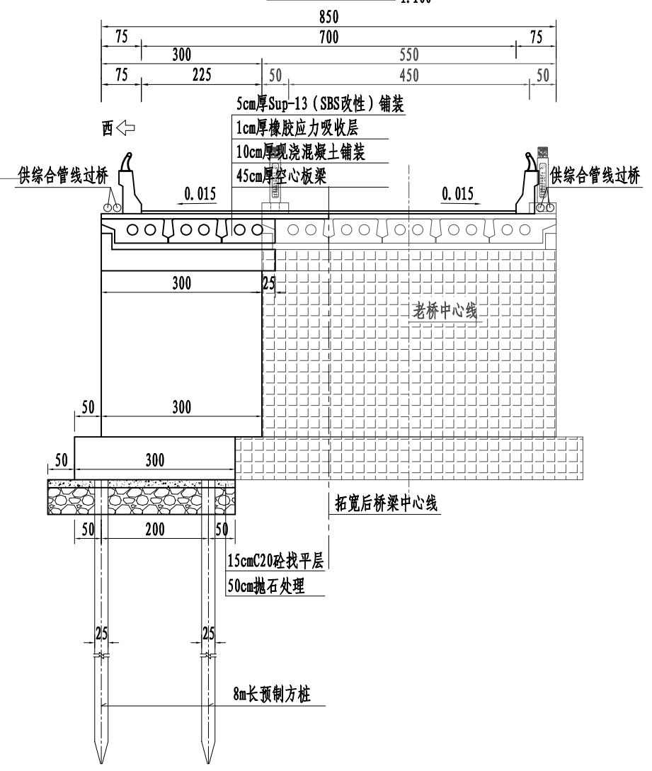
桥台横断面图 1:100
