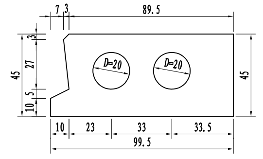
边板 (无挑臂)
