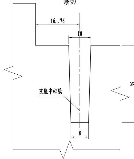
锚栓孔大样
