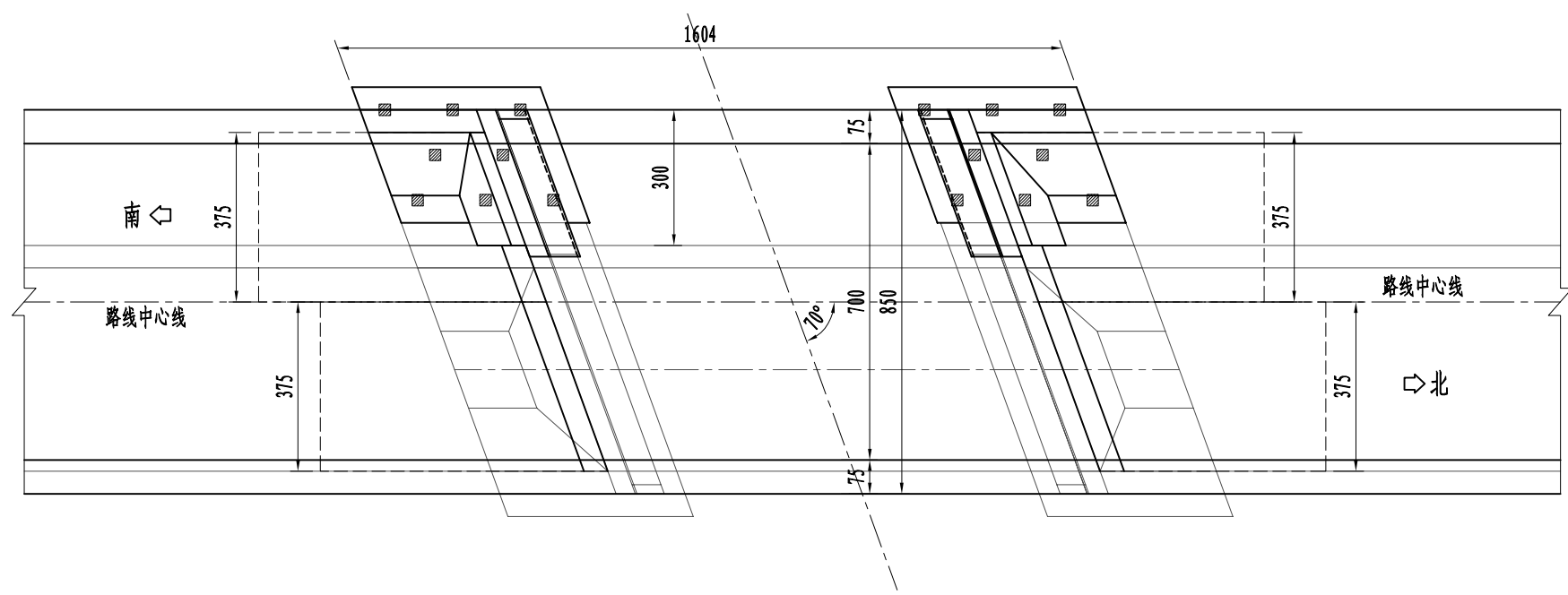
平面 1:150
