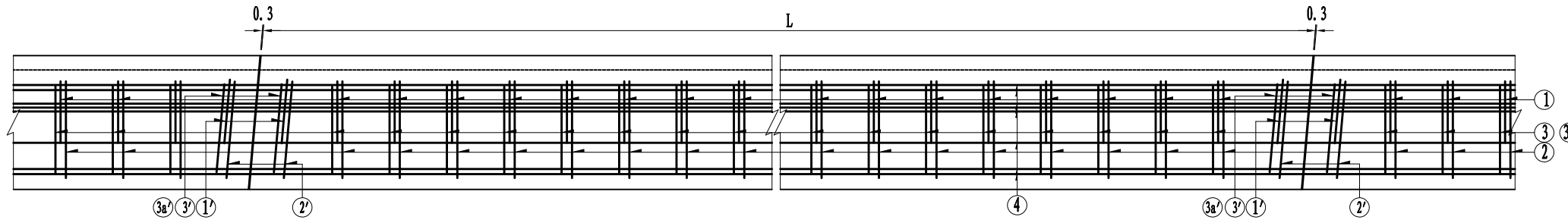
组合式护栏钢筋平面(斜交) 1:20
