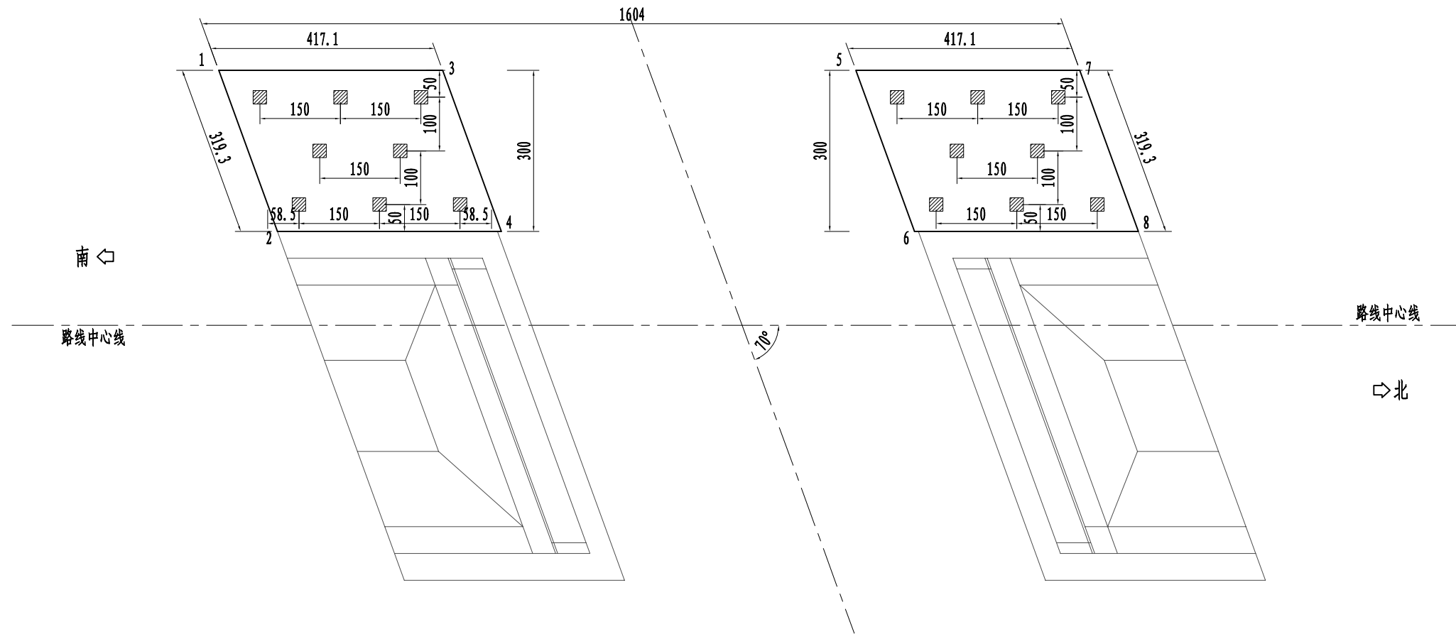
桥台基础编号示意图 1:100
