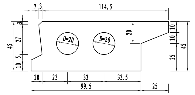
边板 (挑臂25cm)
