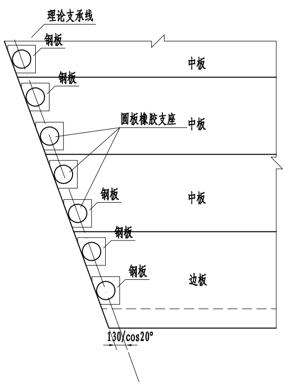
支座安装平面示意
