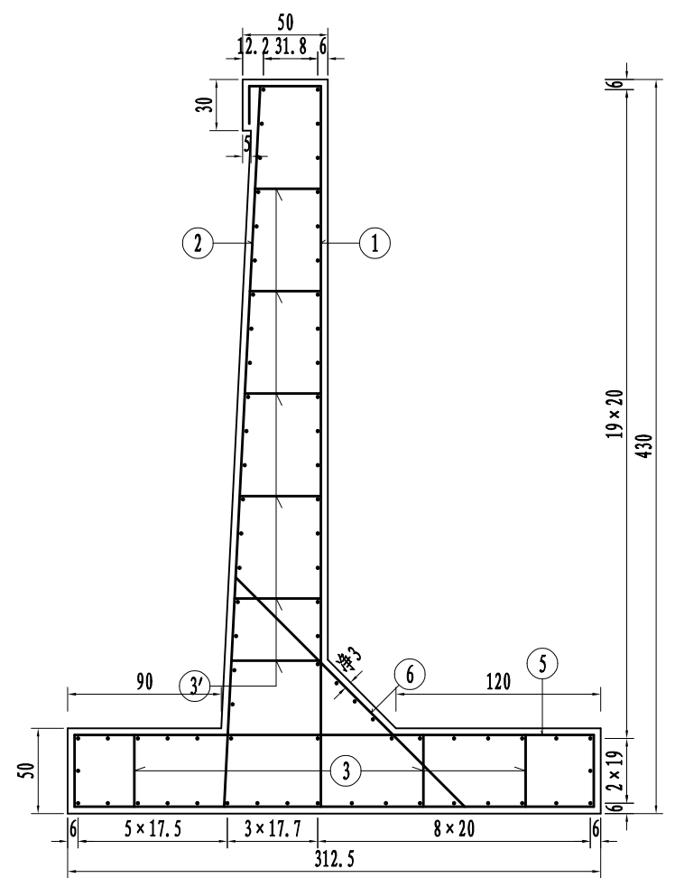
4. 3m高挡墙配筋图 (图中未标示的为4号筋) 1:40
