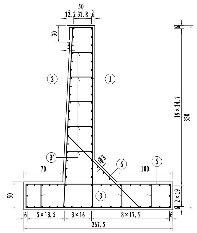
3. 3m高挡墙配筋图 (图中未标示的为4号筋) 1:40
