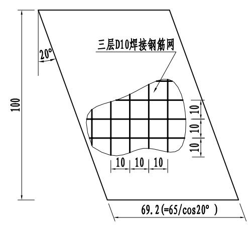
支座垫石平面图 1:20
