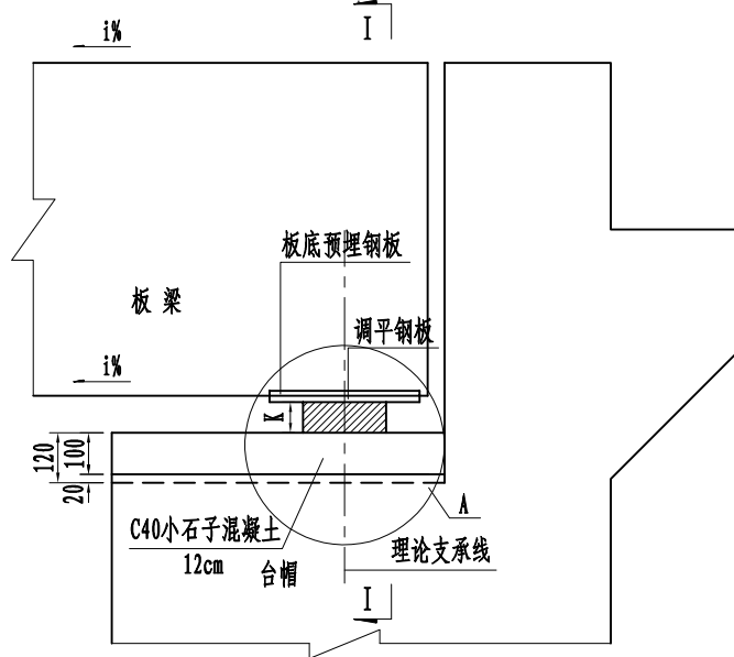
桥台支座安装 (GBZYH(CR)圆板支座) 1:20
