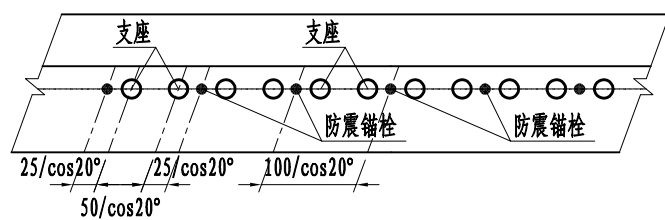
锚栓平面图
