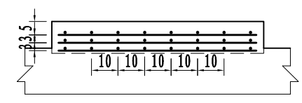
支座垫石断面图 1:20
